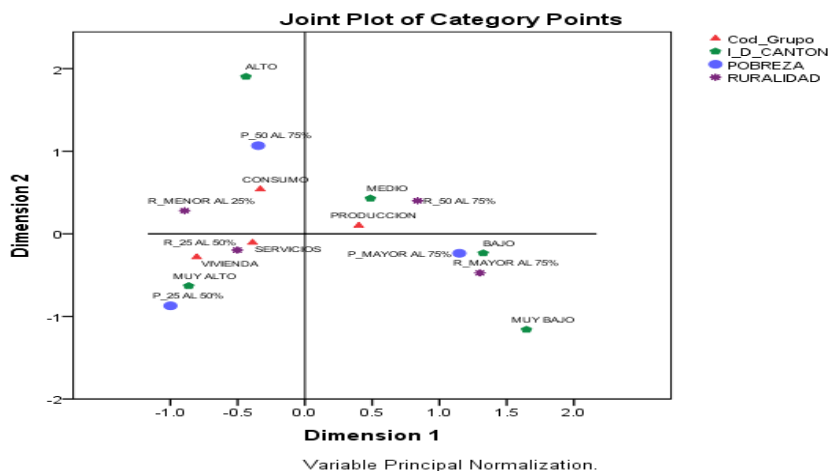
Fig 2. Distribución de las variables en el espacio de los ejes 1 y 2.
